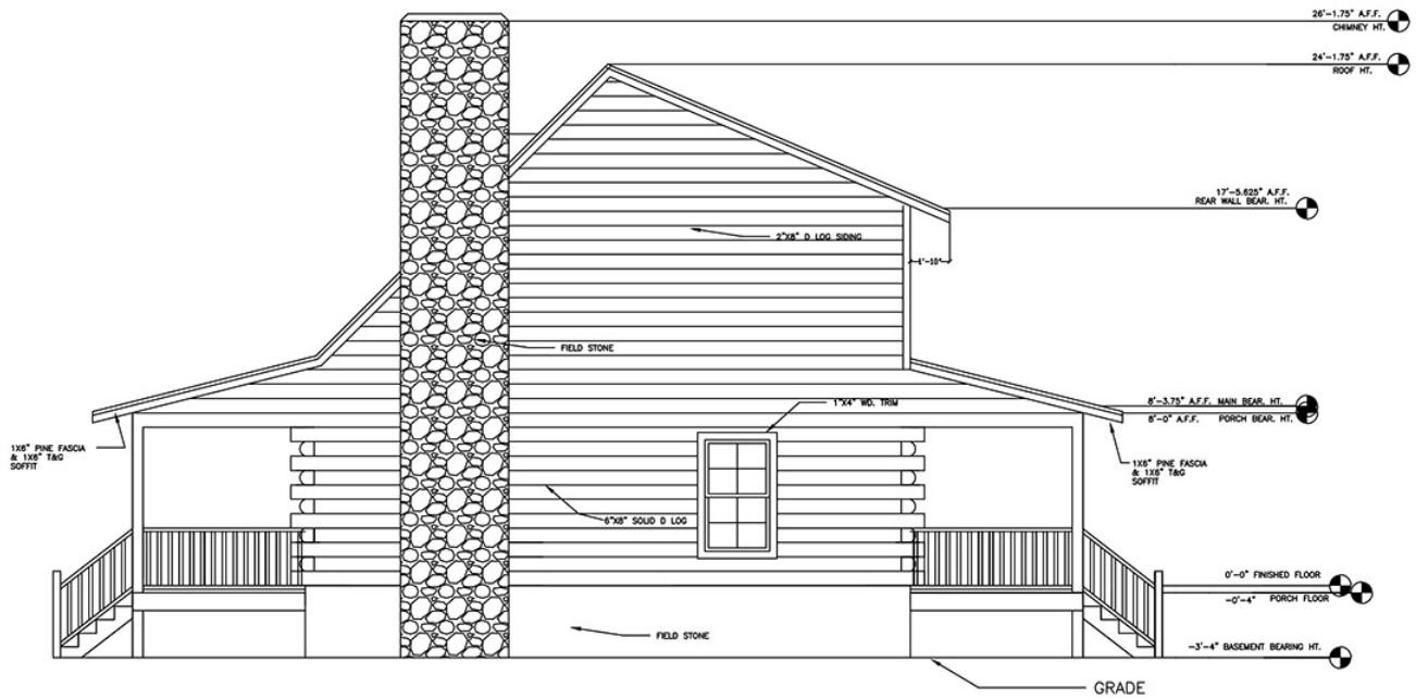
RIGHT ELEVATION
